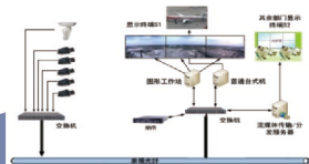
机场全景增强监视系统
